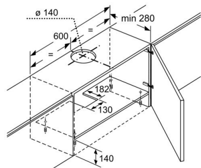
Mõõdud (mm)
