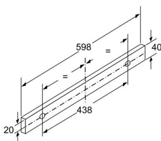
Mõõdud (mm)
