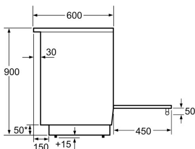
Mõõdud (mm)
