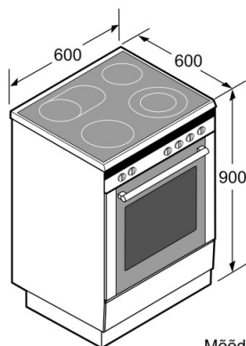
Mõõdud (mm)
