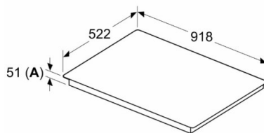
Mõõdud (mm)
