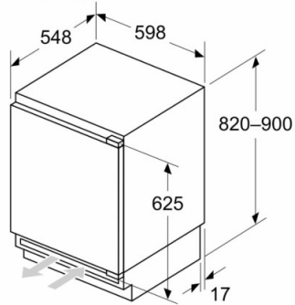
Mõõdud (mm)
