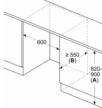
Mõõdud (mm)
