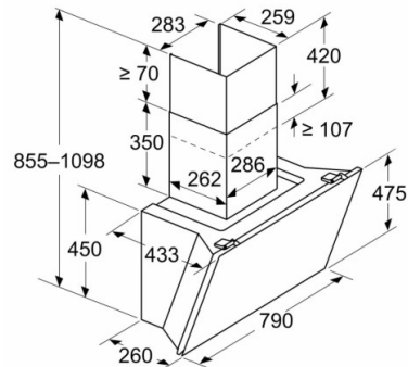
Mõõdud (mm) Seade äratõmberežiimil
