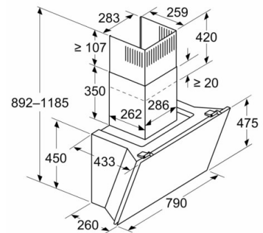
Mõõdud (mm) Seade õhuringlusrežiimil
