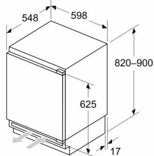
Mõõdud (mm)
