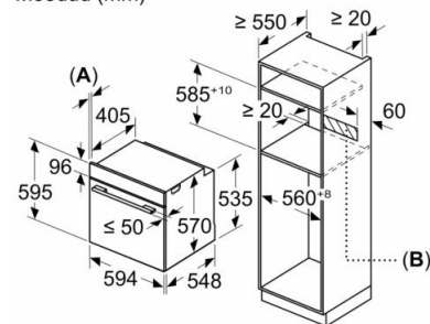
Mõõdud (mm)
