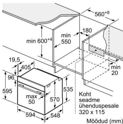
Mõõdud (mm)
