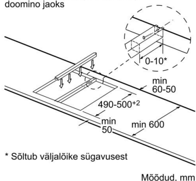
Montaažikomplekt (HEZ394301) domino jaoks
