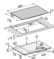
① vorn ② Netzanschlusskasten mit Netzanschlussleitung, L = 1440 mm
