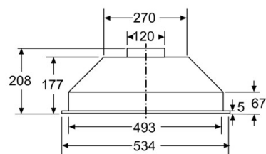
Mõõdud (mm)
