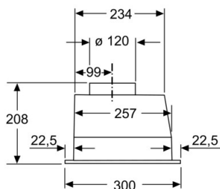
Mõõdud (mm)
