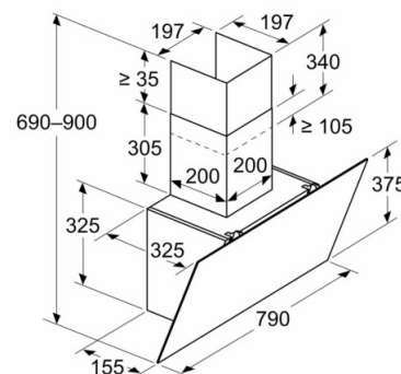
Mõõdud (mm) Seade äratõmberežiimil
