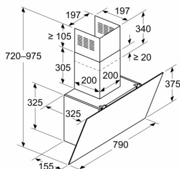
Mõõdud (mm) Seade õhuringlusrežiimil
