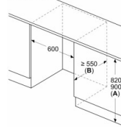
Mõõdud (mm)
