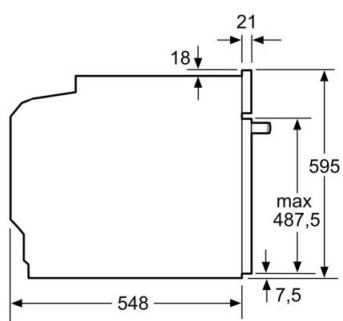
Mõõdud (mm)
