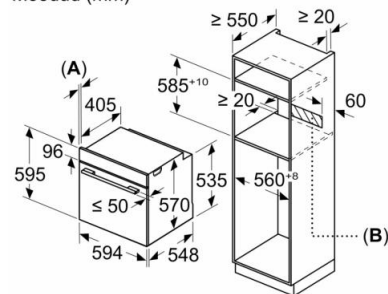
Mõõdud (mm)
